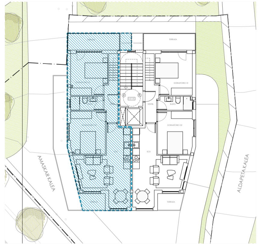
PLANTA TERCERA e: 1/200
